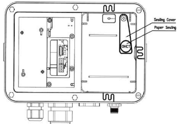
5-6. i-DT33XW Papierdichtung
