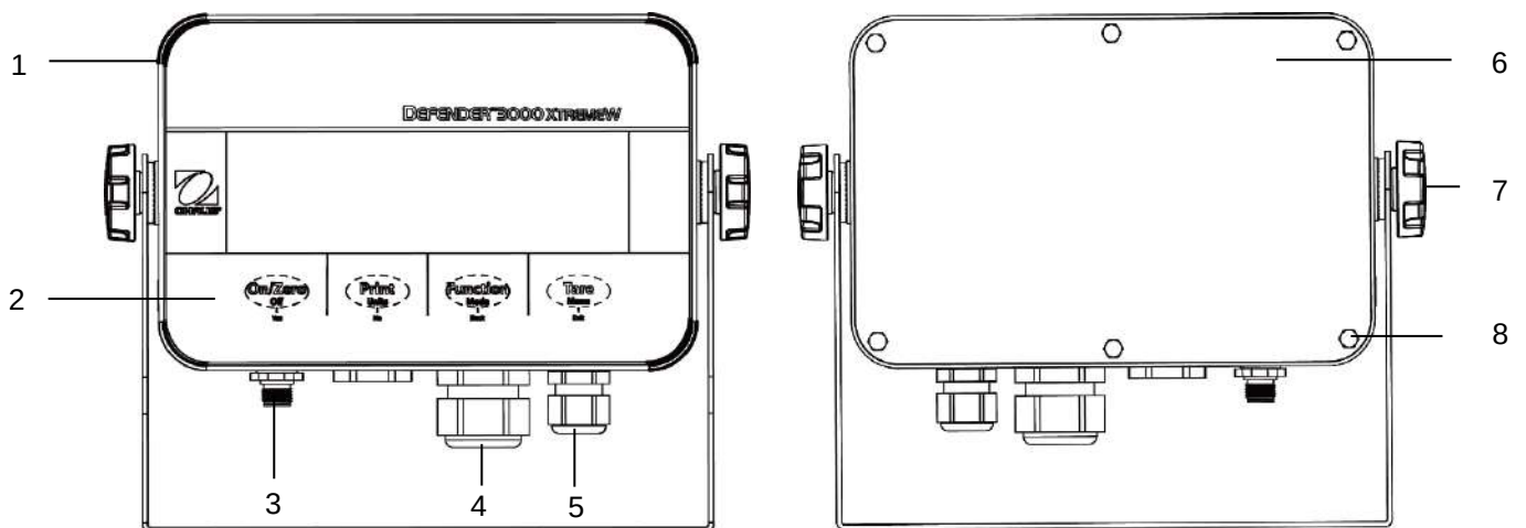
Abbildung 1-2 i-DT33XW Anzeigegerät
