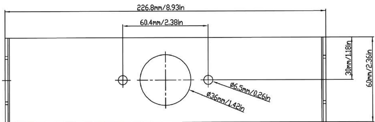
Abbildung 2-8 i-DT33XW Abmessungen der Montagehalterung
