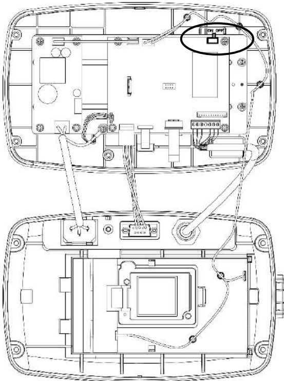
Abbildung 5-1 i-DT33P Position des Sicherheitsschalters (S1)
