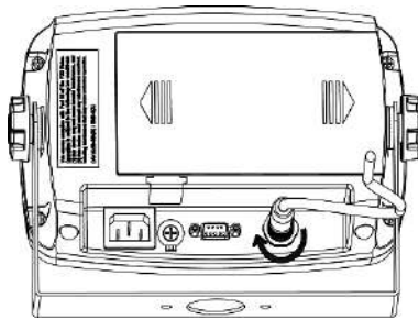
Abbildung 2-1 i-DT33P
