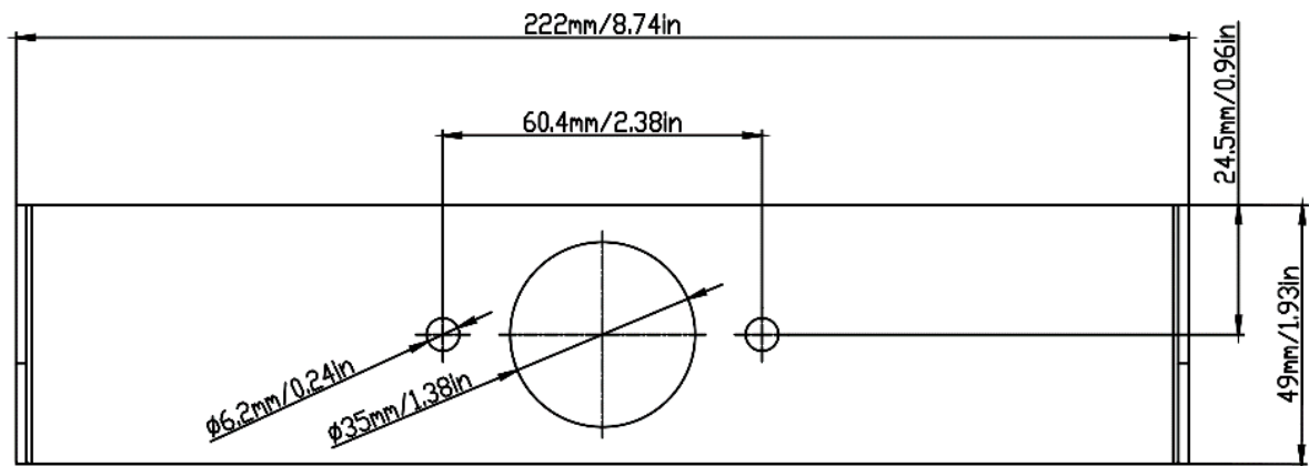
Abbildung 2-7 i-DT33P Abmessungen der Montagehalterung
