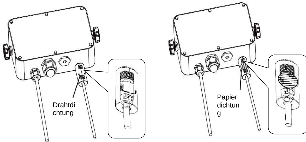
Abbildung 5-9. i-DT33XW Abdichtung (Verbindungskabel mit Anschluss und Speichermodul)
