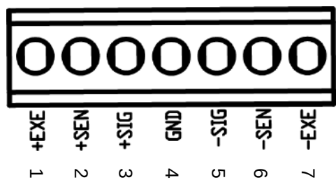
Abbildung 2-3 Wägezellen-Terminalblock
