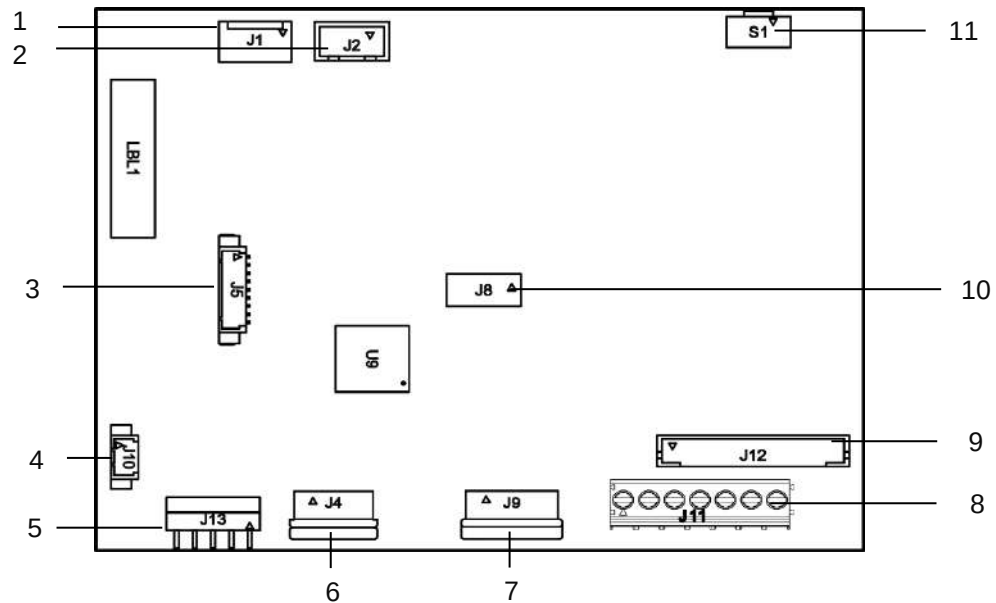
Abbildung 1-3 i-DT33P Mainboard
