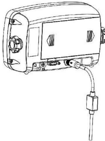
Abbildung 5-7. i-DT33P Abdichtung (Verbindungskabel mit Anschluss und Speichermodul)
