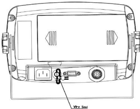
Abbildung 5-3. i-DT33P Drahtdichtung Abbildung
