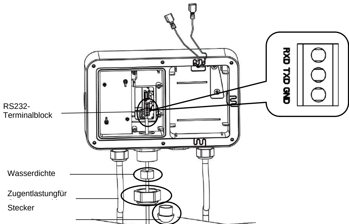
Abbildung 2-6 i-DT33XW RS232-Anschluss
