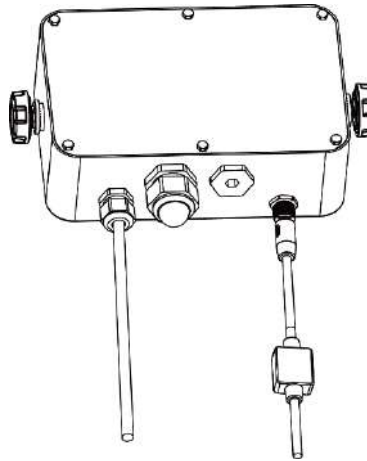
Abbildung 5-9. i-DT33XW Abdichtung (Verbindungskabel mit Anschluss und Speichermodul)
