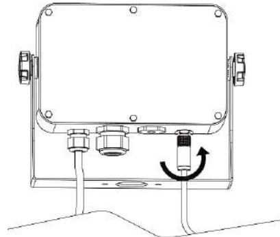
Abbildung 2-2 i-DT33XW
