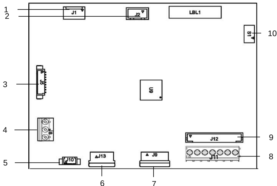
Abbildung 1-4 i-DT33XW Mainboard
