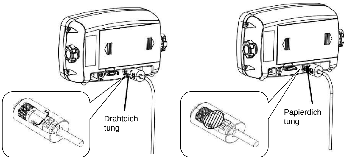
Abbildung 5-8. i-DT33P Versiegelung (Verbindungskabel mit Stecker und ohne Speichermodul)
