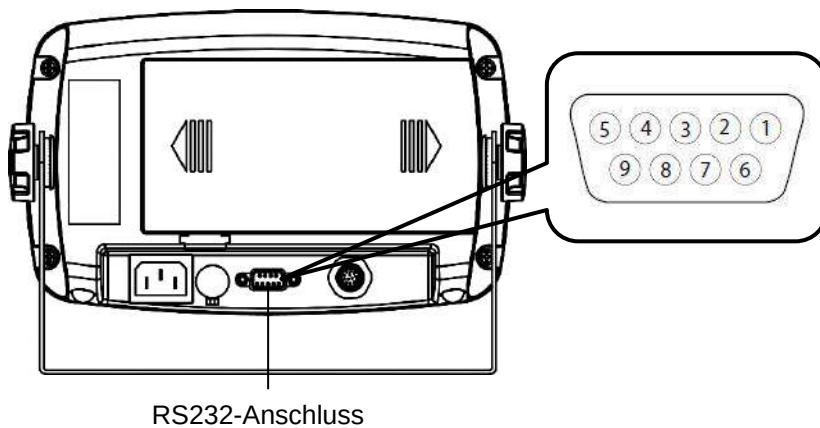
Abbildung 2-5 i-DT33P RS232-
